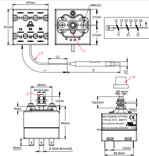
1 : Etalonnage scellé; 2 : Gainage du capillaire; 3 : Bouton de réarmement manuel; 4 : Capuchon du bouton de réarmement
