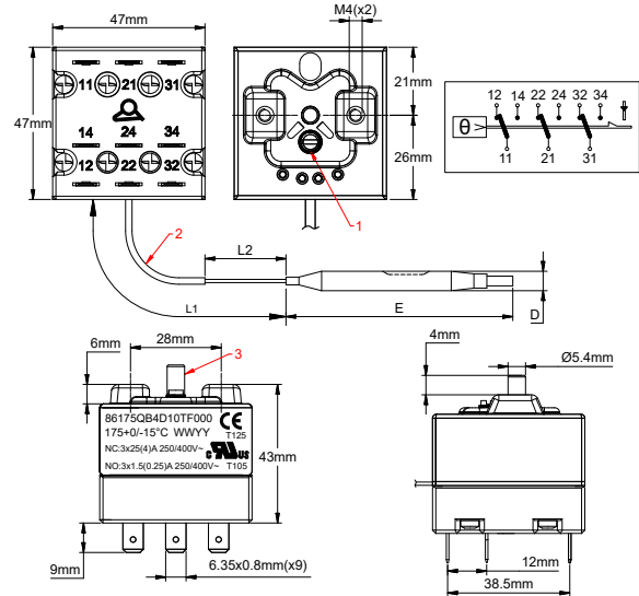
1 : Etalonnage scellé; 2 : Gainage du capillaire; 3 : Bouton de réarmement manuel
