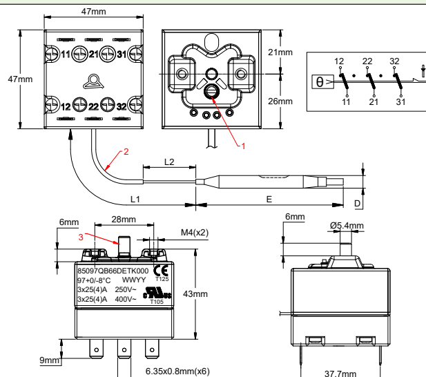
1. Scellé; 2. gainé; 3. Bouton de réarmement manuel
