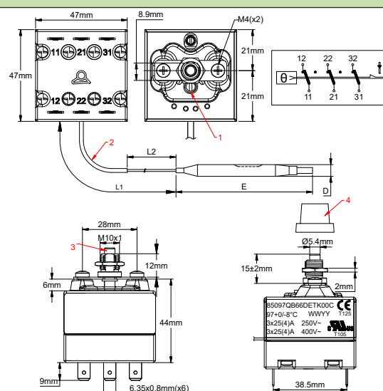
1. Scellé; 2. gainé; 3. Bouton de réarmement manuel; 4. Capuchon plastique (Noir)
